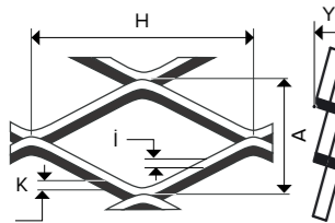
D3 - 1.8 x 3 x 0.5 x 0.45 mm
