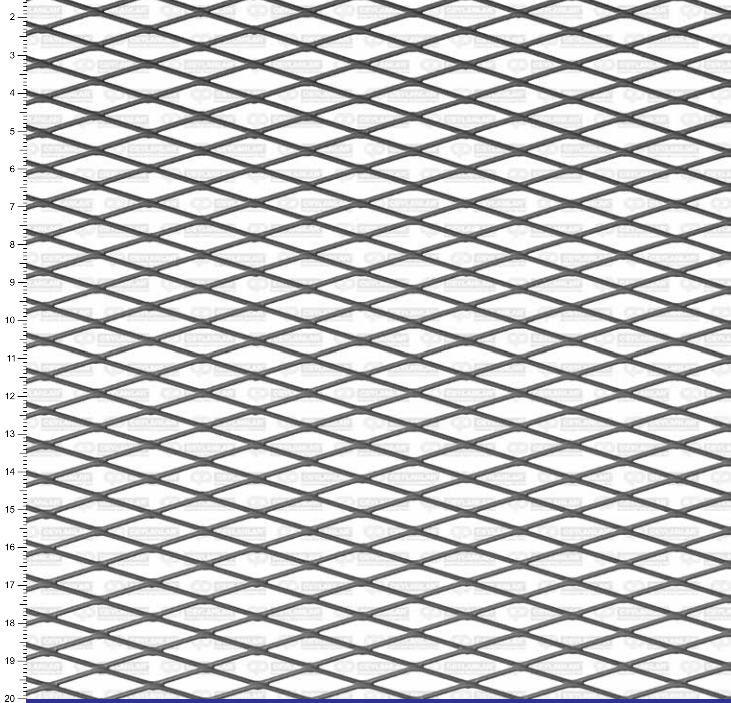
D27 - 9 x 27 x 1 x 1.43 mm
