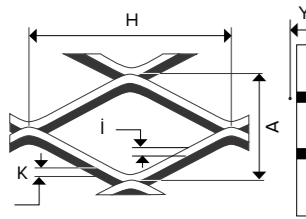
DF42 - 14(16.2) x 42 x 2 x 2.75 mm
