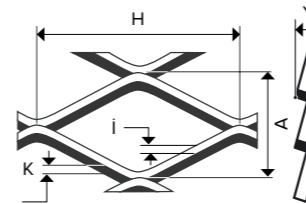
D4 - 2 x 4 x 0.5 x 0.46 mm
