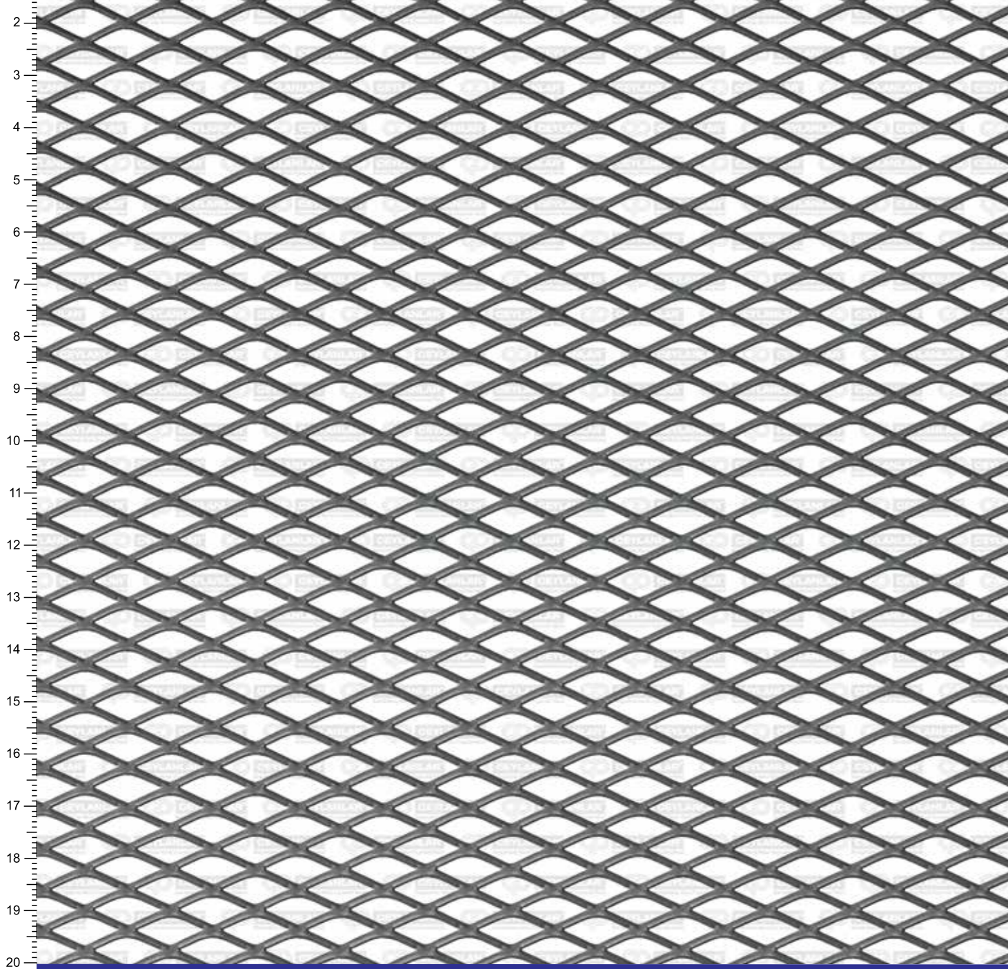
D16 - 8 x 16 x 1 x 1.5 mm
