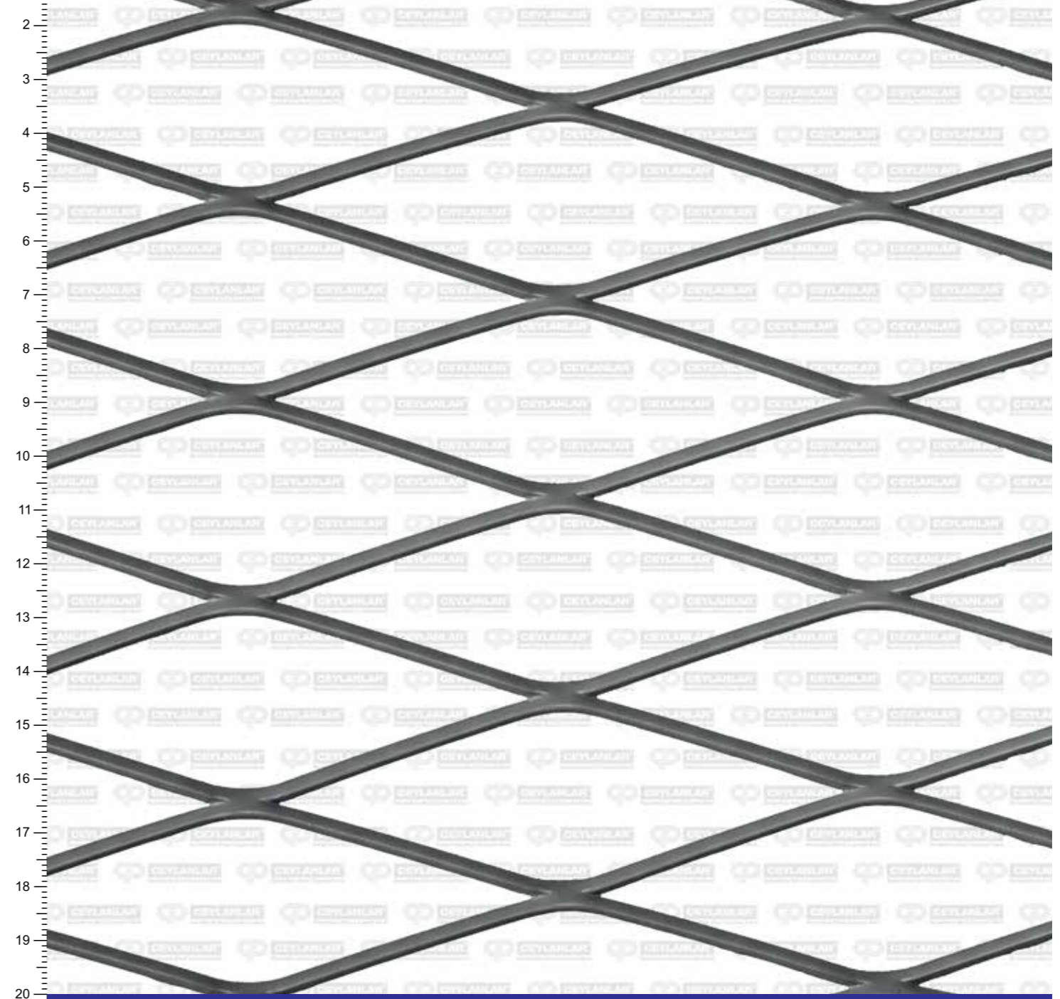
D115 - 40 x 115 x 2 x 3 mm
