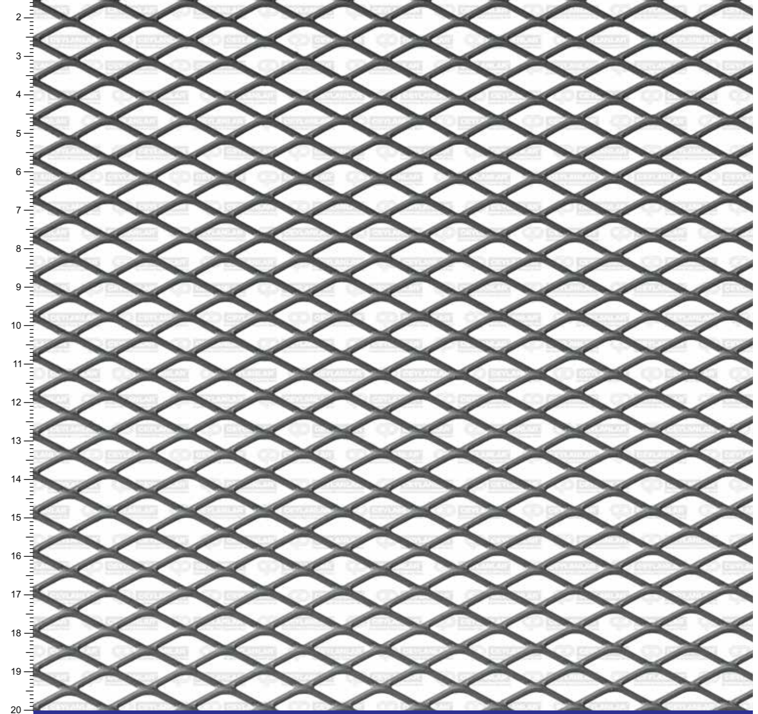
D20-1.5 - 10 x 20 x 1.5 x 1.5 mm
